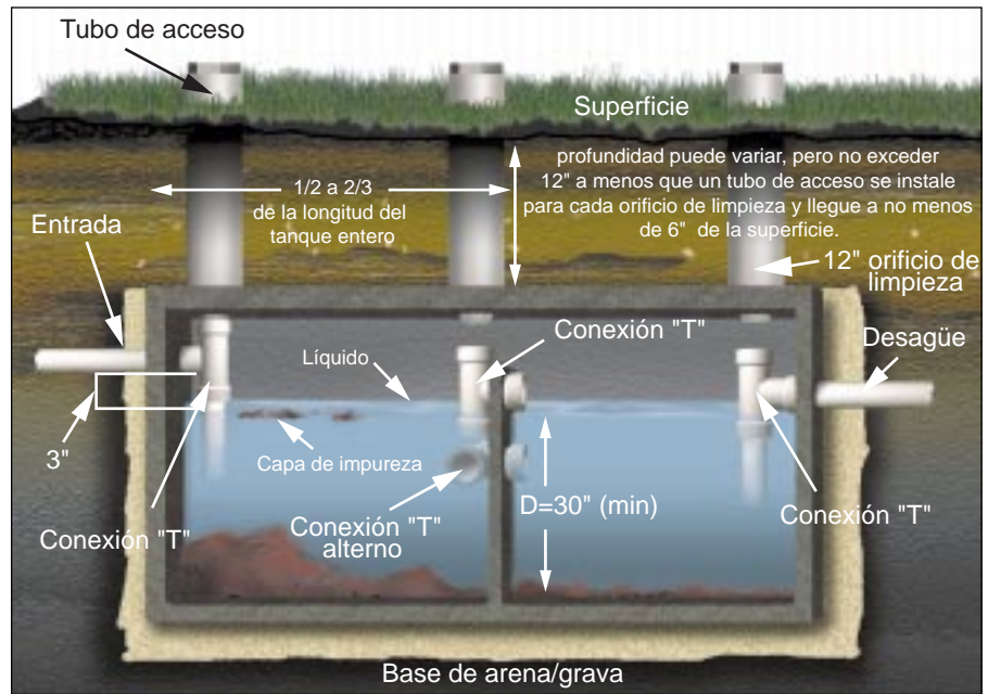
Figura 2: Una fosa séptica de dos compartimientos.
